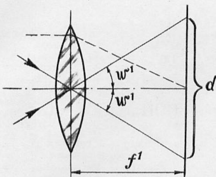
Рис. 1. Поле зрения и фокусное расстояние линзы.
