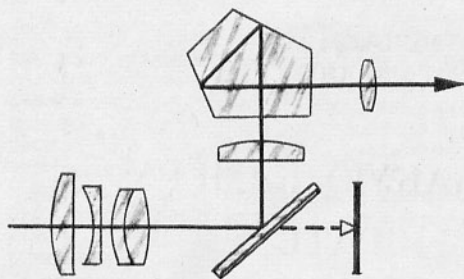
Ход лучей в зеркальной камере.
