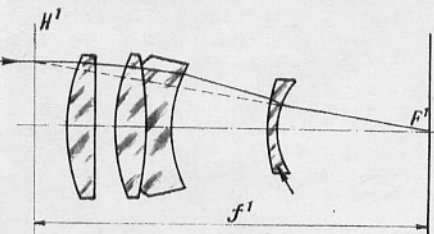
Рис. 5. Схема телеобъектива. Стрелкой показана отрицательная линза.
