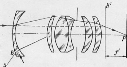
Рис. 4. Схема широкоугольного объектива с увеличенным задним отрезком. Стрелкой показана отрицательная линза.
