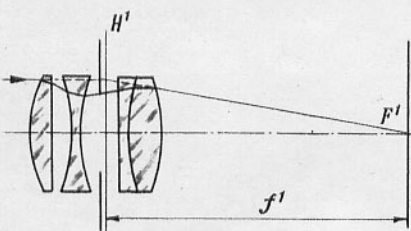
Рис. 3. Нахождение задней главной плоскости объектива.
