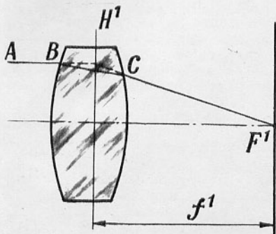
Рис. 2. Нахождение задней главной плоскости линзы H' .
